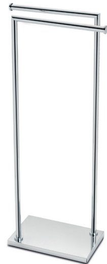
SIMO50 Piantana Porta Salviette - Standing Towel Holder A 5.8300 B 7.0400 L. 30 - H. 83 - P. 18
